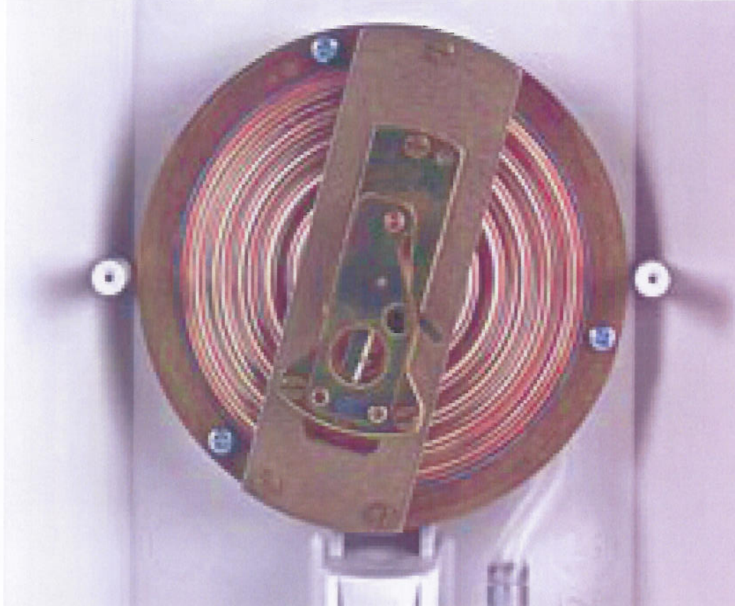
Slika 1: Pričvršćenje preciznog mehanizma na čvrst metalni nosač i tlačna membrana
